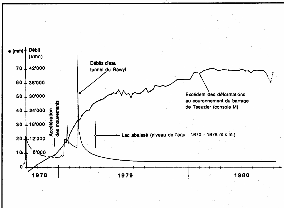
Figure 5 : Comparaison entre l'évolution du débit drainé par le tunnel et le développement des déformations (e) au couronnement du barrage de Tseuzier (d'après BADOUX 1982a). Les pointes de débit correspondent à la rencontre des sources du Synclinal du Lac (2760, 2830, 2860 et 3042). Le début des mouvements de tassement du barrage de Tseuzier s'observe déjà quelques jours seulement après la rencontre de la grosse source 2760 à fin septembre 1978 (environ 13'000 l/mn). Toutefois, une accélération des tassements intervient à partir de fin 1978, sans que de nouvelles venues d'eau soient rencontrées entre-temps. Le ralentissement et la stabilisation des mouvements du barrage coïncident avec la stabilisation du débit drainé par le tunnel.
