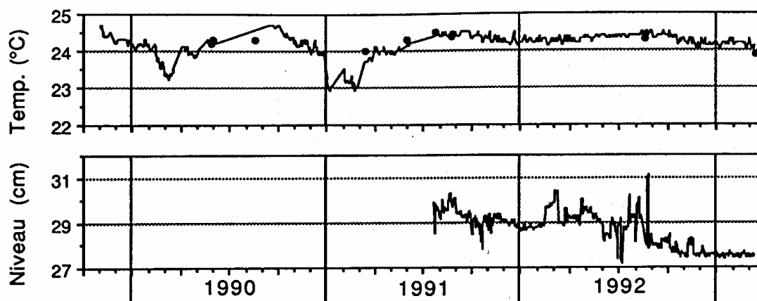
Figure 4 : Evolution de la température et du niveau de l'eau du canal du tunnel au cours de la période novembre 1989 - mars 1993 (relevés MADD). Les mesures ponctuelles manuelles de température sont représentées par des points. Les variations de niveau sont représentatives de l'évolution des débits. Une diminution de la température se produit à deux reprises (hiver 1990 et 1991), mais ne se répète plus en 1992 et 1993. Dans l'ensemble, ces deux paramètres ne présentent pas de variations saisonnières importantes qui pourraient être corrélées avec des phénomènes météorologiques.
