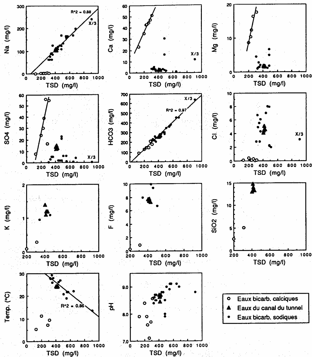
Figure 7 : Comportement des paramètres principaux en fonction de la minéralisation totale (TSD). La plupart des sources représentées n'ont été analysées qu'une seule fois, alors que l'eau du canal l'a été 4 fois. Entre les eaux du tunnel et du forage X/3, de type bicarbonaté-sodique (•), un système de mélange peut être mis en évidence (diagrammes Na/TSD et HCO 3 /TSD). Le pôle faiblement minéralisé est représenté par les eaux les plus chaudes, qui proviennent des calcaires fissurés et karstifiés du Malm. Les eaux du pôle plus minéralisé sont les moins chaudes et proviennent des formations marno-calcaires du Dogger. Sur le diagramme HCO 3 /TSD, les eaux froides de type bicarbonaté-calcique (○) et les eaux subthermales et thermales de type bicarbonaté-sodique (•) s'alignent sur une même droite de corrélation. Cette observation tend à démontrer que toutes ces eaux ont une origine commune.
