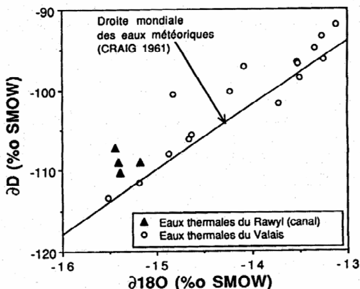
Figure 9 : Deutérium et oxygène-18 dans les eaux du canal comparé à d'autres eaux thermales du Valais (BIANCHETTI, en préparation). Les eaux thermales du tunnel du Rawyl ne s'alignent pas parfaitement sur la droite mondiale des eaux météoriques.
