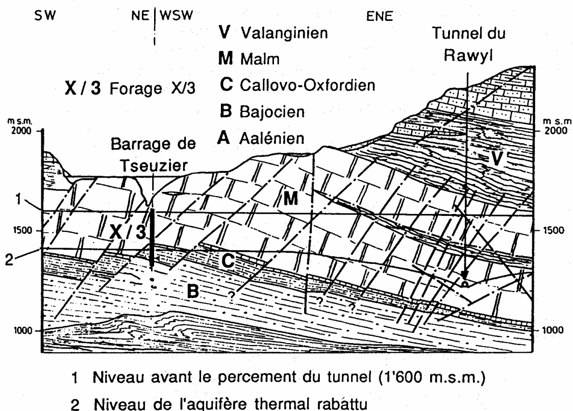
Figure 10 : Profil géologique entre le barrage de Tseuzier et le tunnel, avec situation du forage X/3 (d'après SCHNEIDER 1982). Le tunnel et le forage X/3 ont drainé des eaux bicarbonatées sodiques sous pression provenant d'un même aquifère captif. Les niveaux statiques hypothétiques de la nappe thermique captive avant (1) et après le percement du tunnel (2) ont été représentés.
