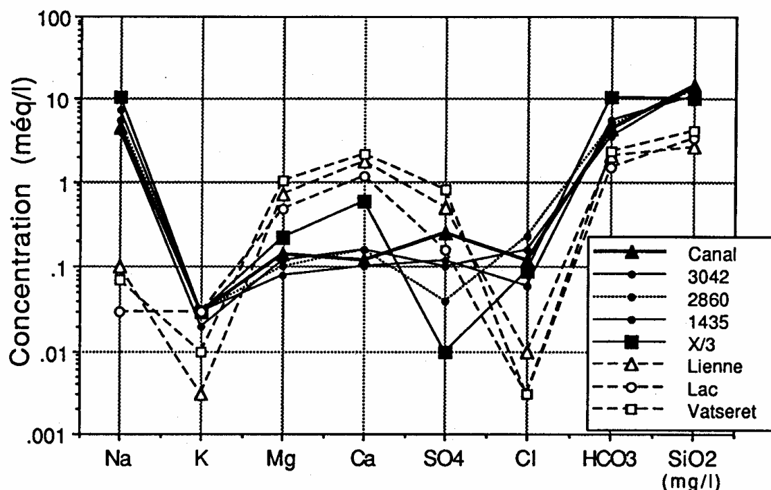
Figure 6 : Représentation avec diagramme de Schoeller de la concentration des ions principaux et de la silice des eaux du tunnel et de la région. Les eaux du tunnel et du forage X/3, dont la minéralisation dépend presque entièrement du sodium et du bicarbonate, se distinguent nettement des eaux froides de l'aquifère karstique de l'Urgonien et des eaux de surface (torrent Lienne, lac de Tseuzier et source de Vatseret). Les eaux bicarbonatées-sodiques thermales représentent probablement une évolution par échange cationique des eaux bicarbonatées-calciques.
