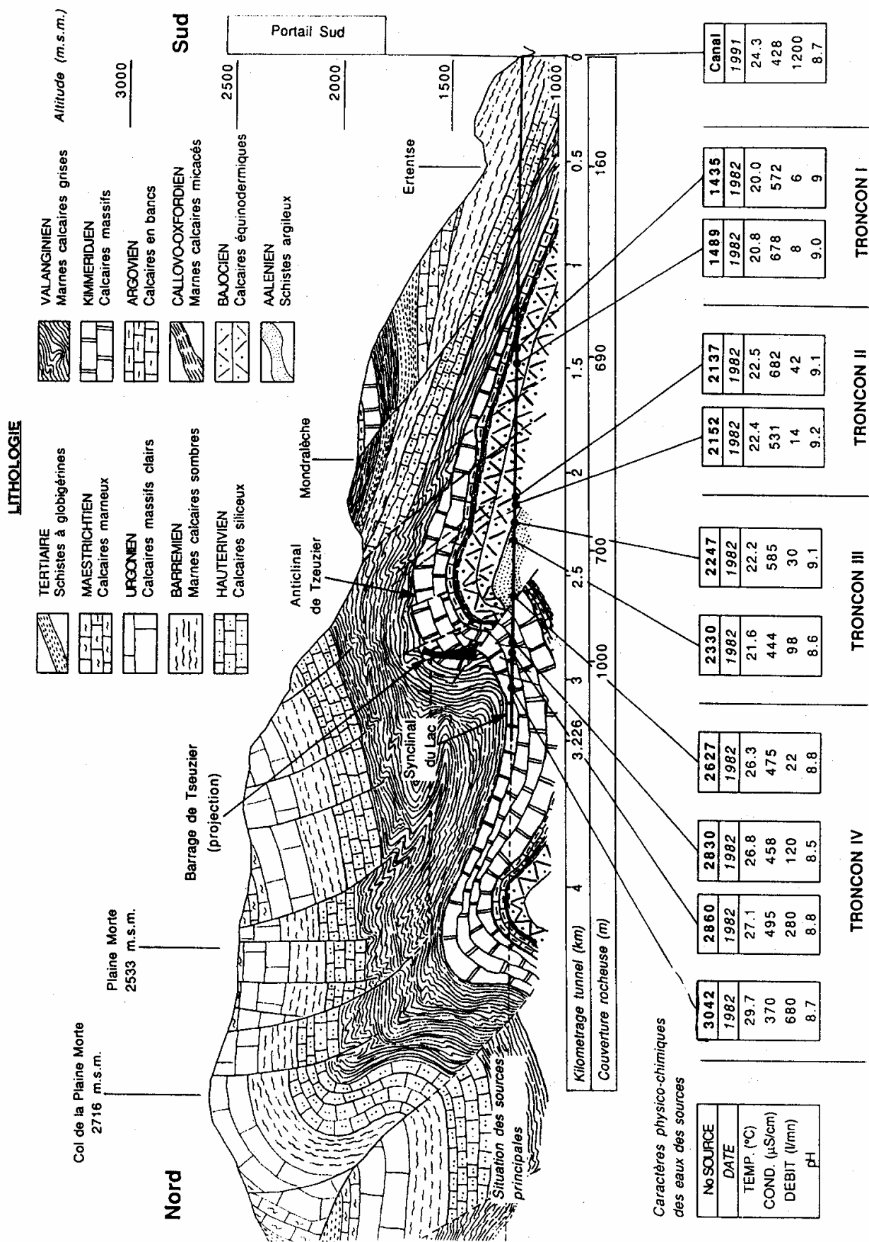
Figure 3 : Profil géologique du tunnel (modifié d'après BADOUX 1982a), avec situation et principales caractéristiques physico-chimiques des venues d'eau.
