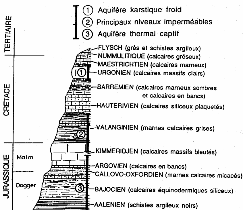
Figure 2 : Coupe litho-stratigraphique "type" de la nappe du Wildhorn (d'après SCHNEIDER 1982). Des formations calcaires compétentes alternent avec des formations marneuses. Les principales circulations d'eau s'observent dans les calcaires karstifiés de l'Urgonien (aquifère karstique froid) et dans les calcaires fissurés du Malm (aquifère thermal captif). Les marnes du Barrémien, du Valanginien et du Callovo-Oxfordien, ainsi que les schistes argileux de l'Aalénien représentent les aquicludes.
